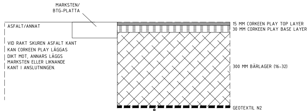
ANSLUTNING CORKEEN PLAY MOT HÅRDGJORDA YTOR TYP ASFALT, BETONGMARKSTEN M.M. SKALA 1:10
