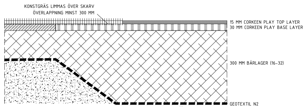
DOLD KANT CORKEEN PLAY MOT KONSTGRÄS SKALA 1:10
