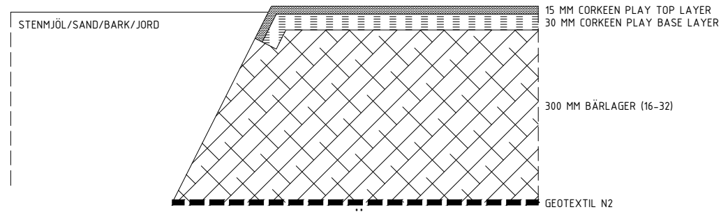
ANSLUTNING CORKEEN PLAY MOT LÖSA MATERIAL TYP STENMJÖL, SAND, BARK M.M. SKALA 1:10
